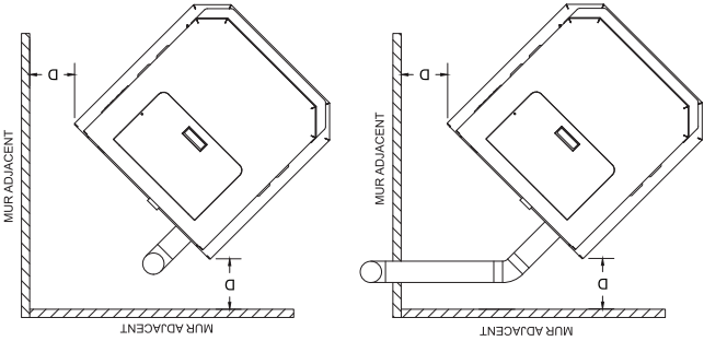
FIGURE 4 DÉGAGEMENT AVEC LE MUR LATÉRAL EN CAS D'INSTALLATION EN COIN
