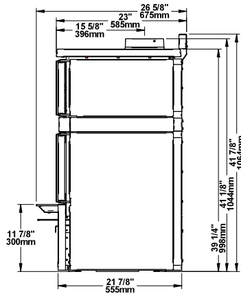
CUISINIÈRE À BOIS GUSTO (OB02047)
