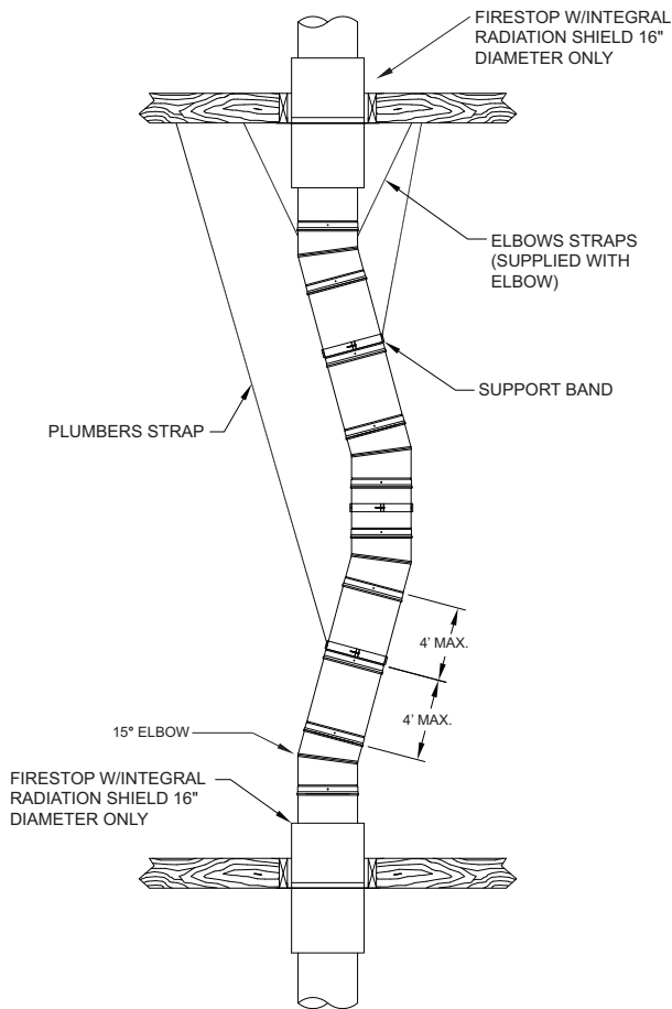
FIG. 12B (16" Diameter)
