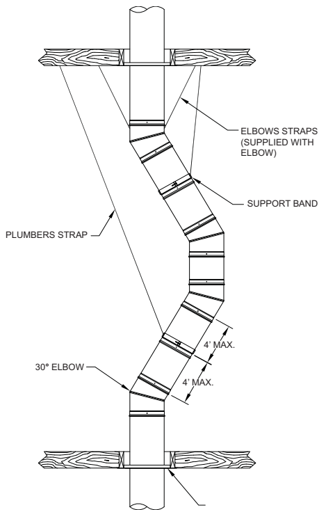
FIG. 12A (8"-14" Diameters)
